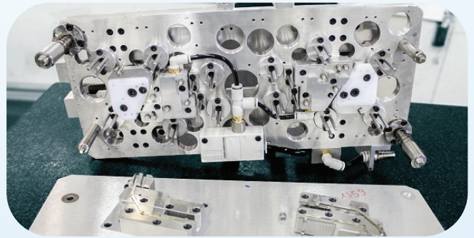
ĐỒ GÁ JIG CHUYÊN DỤNG
