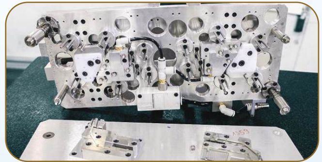
ĐỒ GÁ JIG CHUYÊN DỤNG Specialized JIG
